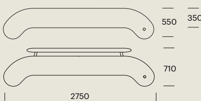
#193 PLINTH #194 WALL-BENCH
