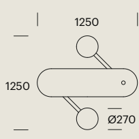
#193 PLINTH #194 WALL-BENCH
